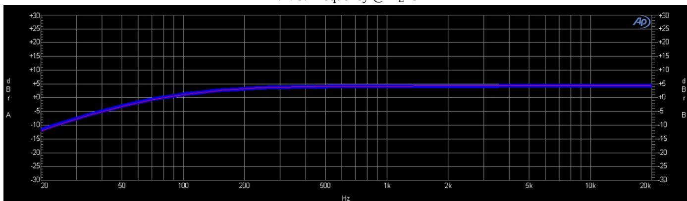
Av VS. Frequency @ R_L=32\Omega
