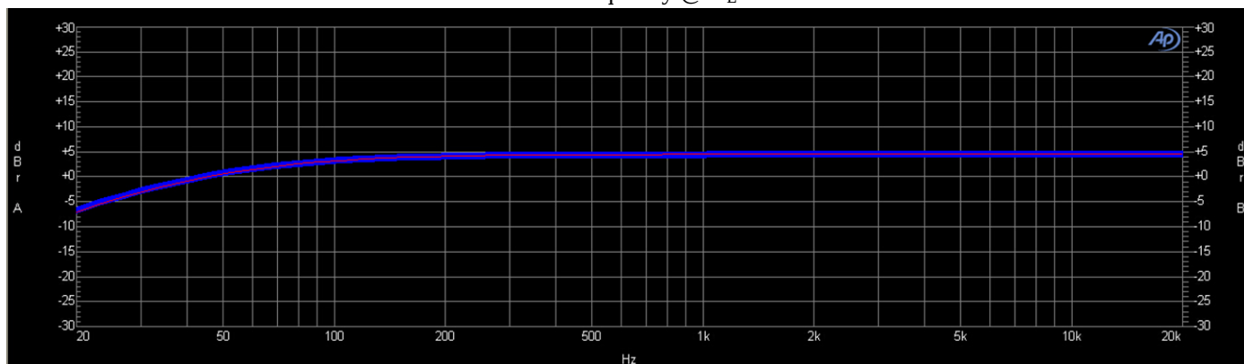
Av VS. Frequency @ R_L=16\Omega
