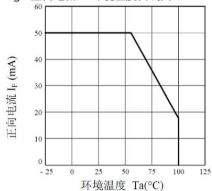
Fig.1 正向电流 vs 环境温度曲线图
