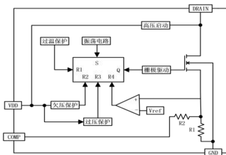
图 1 电路功能框图
